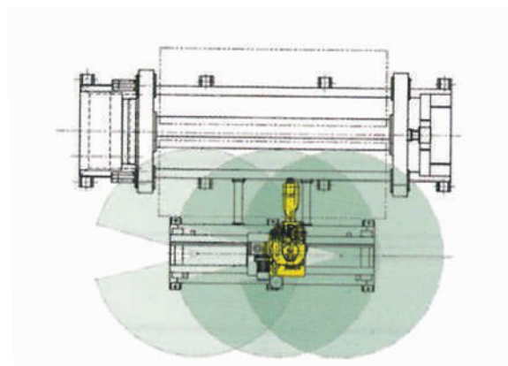
Cella egy robottal
